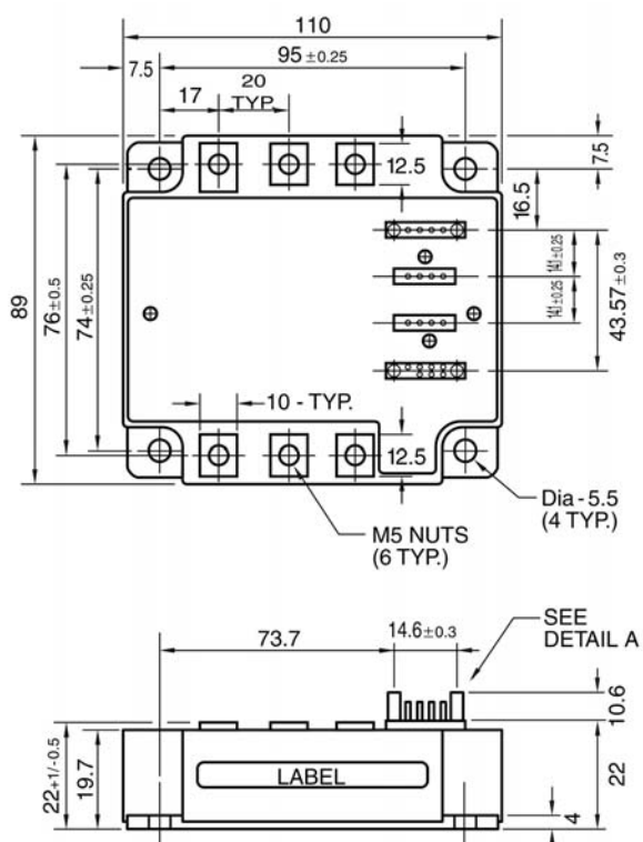
Package V5
