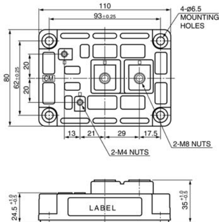
Package A5
