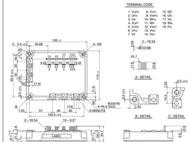
Package S8
