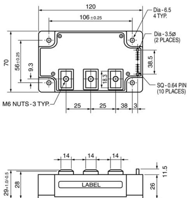
Package V1
