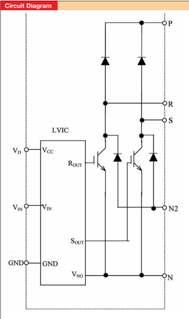
Package D11
