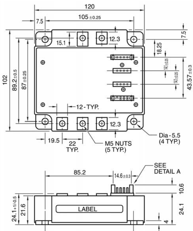
Package V3
