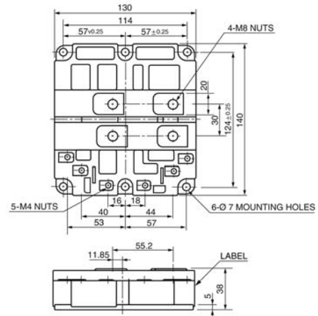
Package HV2
