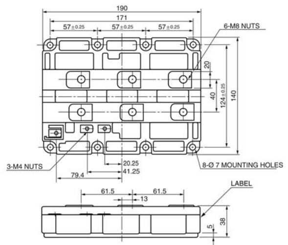
Package HV6
