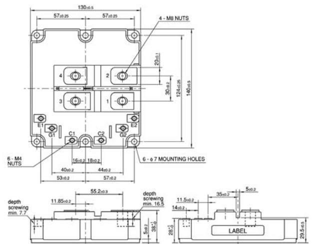
Package HV10
