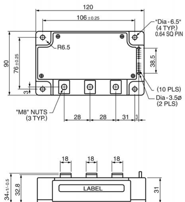
Package V2
