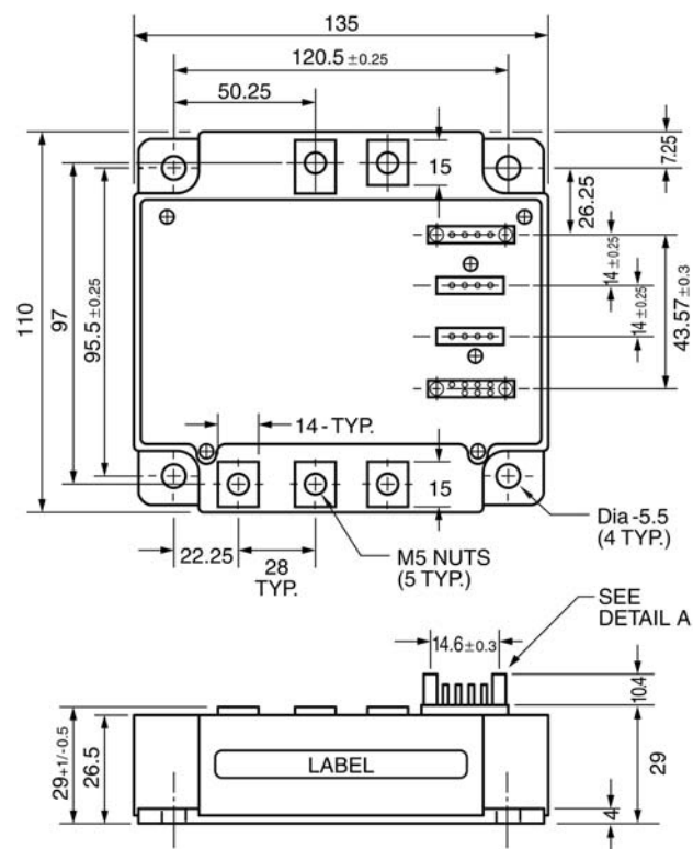
Package V4
