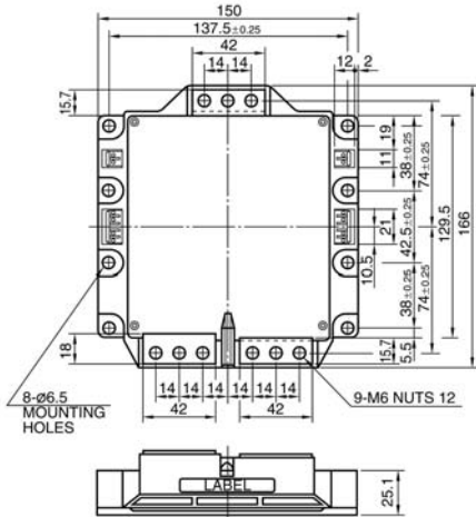
Package MPD1
